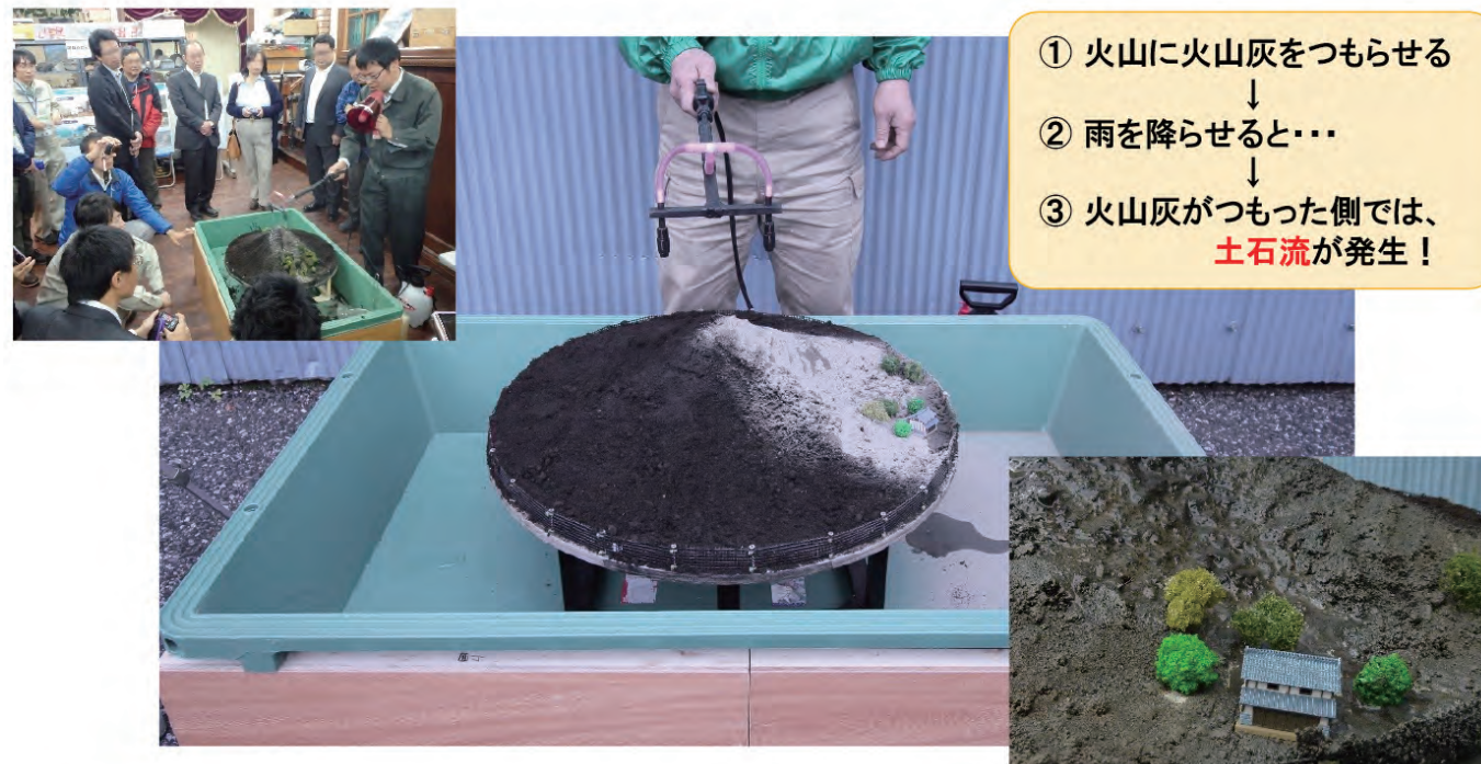
国土交通省九州地方整備局 九州技術事務所における実験状況
